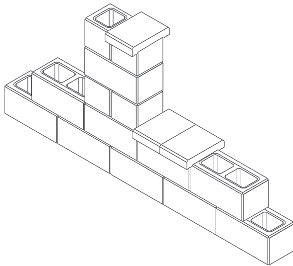
Pustak cały - rozszczepiany z trzech stron
