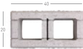
Pustak podmurówkowy - rozszczepiany z dwóch stron
