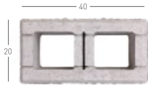
Pustak cały - rozszczepiany z trzech stron
